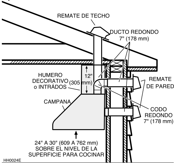
HH0024E CONDUCTOS TÍPICOS DE MODELO H325B CON 1 VENTILADOR
