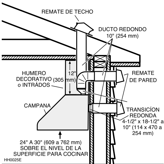
HH0025E CONDUCTOS TÍPICOS DEL MODELO H326B CON 2 VENTILADORES
